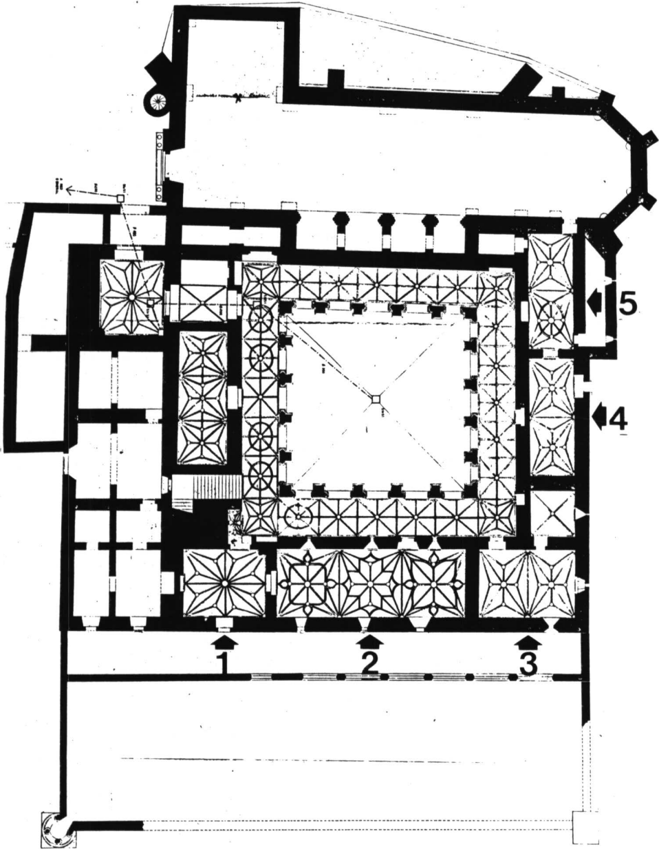
Planta de la Conventual de Calera de León, según el arquitecto José R. Zorita Carrera. Las flechas indican las bóvedas que Byne pretendió desmontar y trasladar a California.
