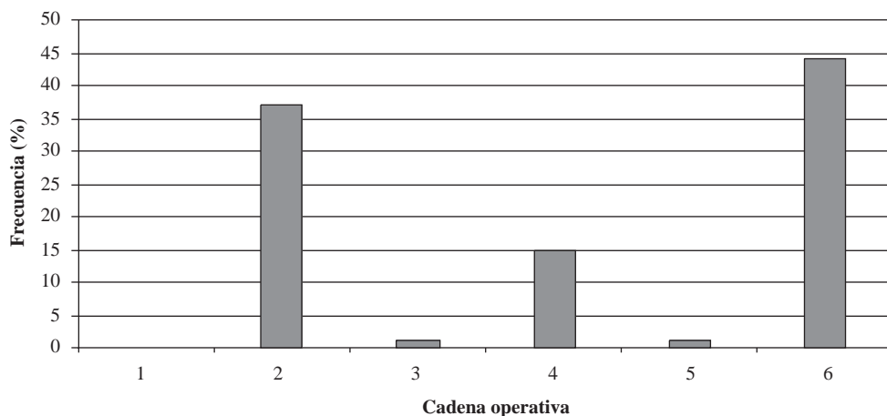
FIGURA 10 FRECUENCIA DE USO DE LAS DISTINTAS CADENAS OPERATIVAS EN LA PRODUCCIÓN DE OBJETOS DE COBRE Y BRONCE DEL BRONCE MEDIO. 1 FUNDICIÓN; 2 FUNDICIÓN+FORJA EN FRÍO; 3 FUNDICIÓN+RECOCIDO; 4 FUNDICIÓN+FORJA EN FRÍO+RECOCIDO; 5 FUNDICIÓN+RECOCIDO+FORJA EN FRÍO; 6 FUNDICIÓN+FORJA EN FRÍO+RECOCIDO+FORJA EN FRÍO.
