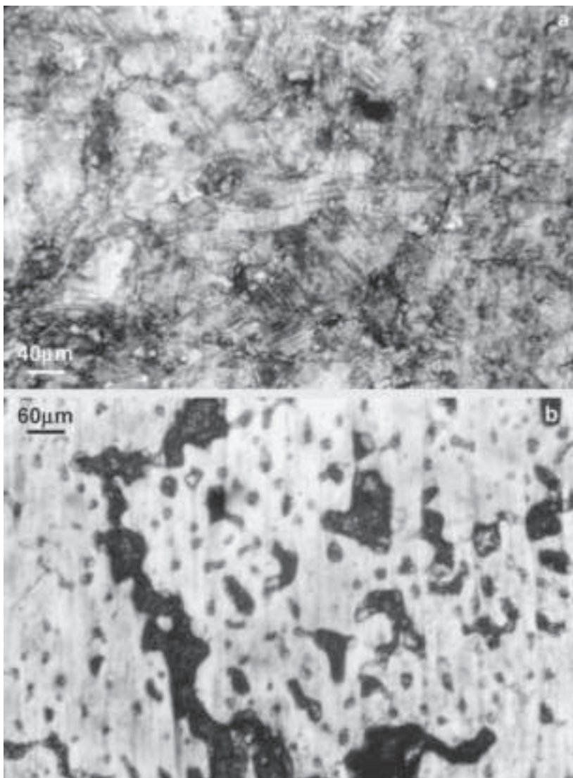
FIGURA 14 METALOGRAFÍAS DE UN HACHA DE TALÓN Y ANILLAS DEL DEPÓSITO DE VARA (LUGO). A) FILO; B) TALÓN. EXPLICACIÓN EN EL TEXTO.
