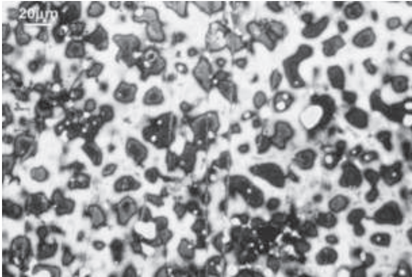
FIGURA 11 MICROESTRUCTURA METALOGRAFICA DE BRUTO DE COLADA DE UN LINGOTE PLANOCONVEXO DE COBRE DEL BRONCE FINAL. LOS NÓDULOS BLANCOS SON IMPUREZAS DE SULFURO DE COBRE.
