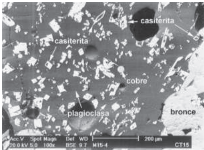
FIGURA 13 SECCIÓN DE UNA ESCORIA DE PRODUCCIÓN DE BRONCE POR REDUCCIÓN CONJUNTA DE MINERALES DE COBRE Y DE ESTAÑO. EXPLICACIÓN EN EL TEXTO.
