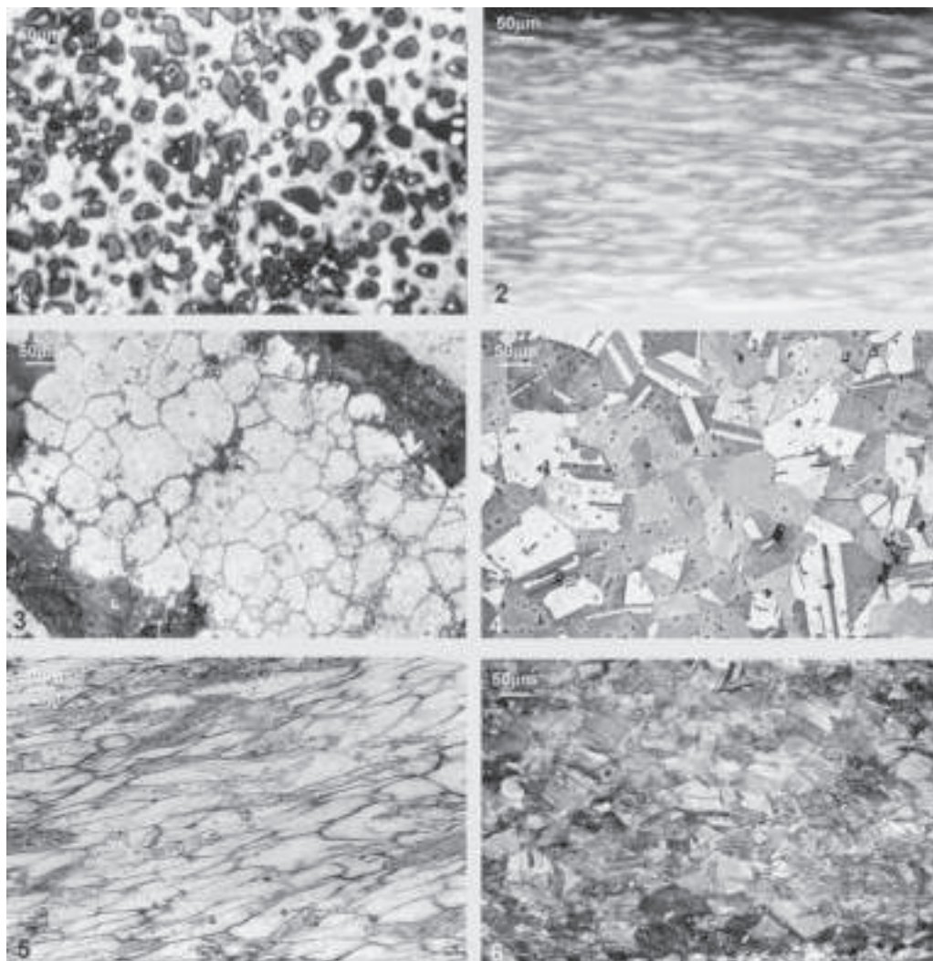
FIGURA 5 SERIE DE MICROESTRUCTURAS METALGRÁFICAS BÁSICAS CORRESPONDIENTES A LAS SEIS CADENAS OPERATIVAS DESCRITAS EN EL TEXTO. IMÁGENES TOMADAS EN EL MICROSCOPIO ÓPTICO.
