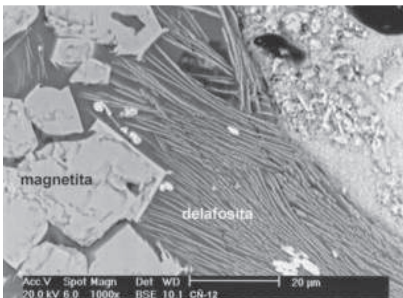
FIGURA 3 DETALLE DE UNA FORMACIÓN DE DELAFOSITA Y MAGNETITA EN LA CAPA DE ESCORIA DE UNA VASIJA DE REDUCCIÓN. IMAGEN VISTA EN EL MICROSCOPIO ELECTRÓNICO DE BARRIDO.
