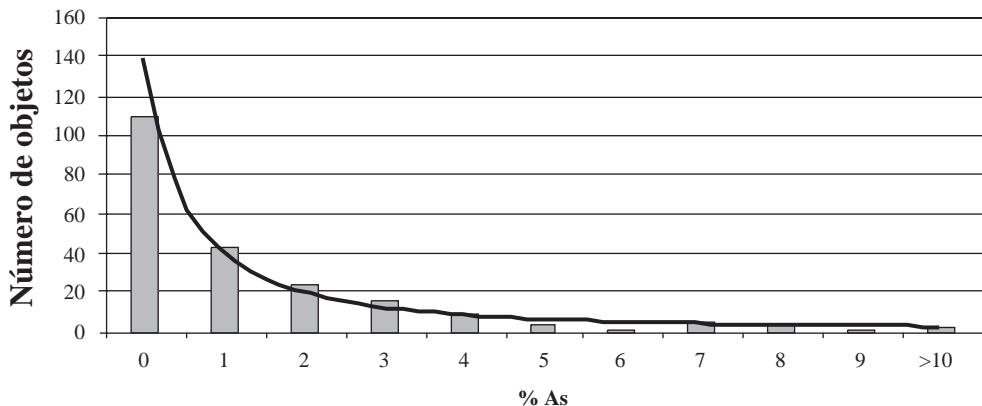
FIGURA 4 CONTENIDO DE ARSÉNICO EN LOS OBJETOS DE COBRE DE LA CULTURA DE LOS MILLARES.
