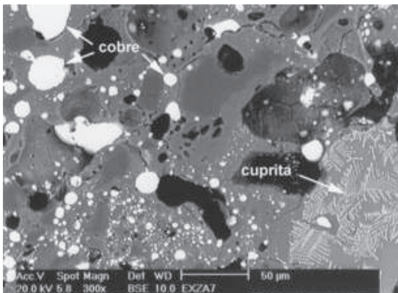
FIGURA 1 ESCORIA EXPERIMENTAL DE COBRE VISTA EN EL MICROSCOPIO ELECTRÓNICO DE BARRIDO. LAS MASAS Y BOLITAS BLANCAS SON COBRE METÁLICO.
