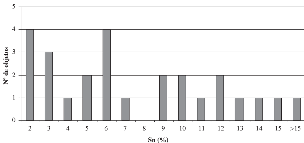
FIGURA 9 CONTENIDO DE ESTAÑO EN LOS BRONCES ARGÁRICOS.
