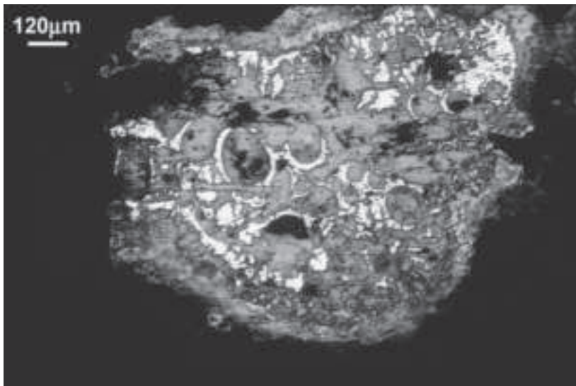
FIGURA 12 SECCIÓN METALOGRAFICA DE UN NODULILLO METÁLICO DE PEÑA NEGRA (CREVILLENTE, ALICANTE). EXPLICACIÓN EN EL TEXTO.
