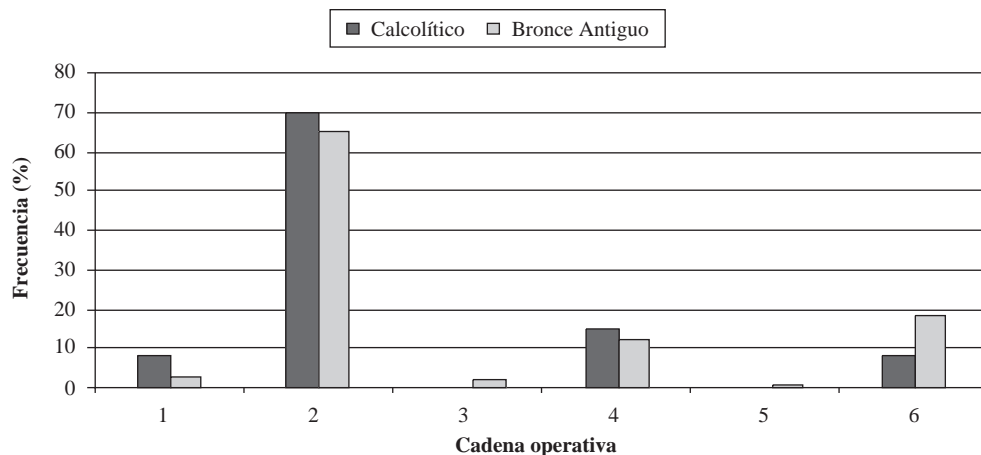
FIGURA 6 FRECUENCIA DE USO DE LAS DISTINTAS CADENAS OPERATIVAS EN LA PRODUCCIÓN DE OBJETOS DE COBRE CALCOLÍTICOS Y DEL BRONCE ANTIGUO. 1 FUNDICIÓN; 2 FUNDICIÓN+FORJA EN FRÍO; 3 FUNDICIÓN+RECOCIDO; 4 FUNDICIÓN+FORJA EN FRÍO+RECOCIDO; 5 FUNDICIÓN+RECOCIDO+FORJA EN FRÍO; 6 FUNDICIÓN+FORJA EN FRÍO+RECOCIDO+FORJA EN FRÍO.
