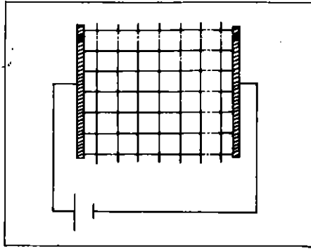
Figura 1: Esquema simplificado del experimento de Watson y Leath.
