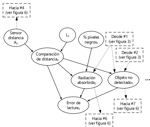
Figura 4: Detección de errores sistemáticos para la subred de anomalías correspondiente al rayo #2 del telémetro láser.
