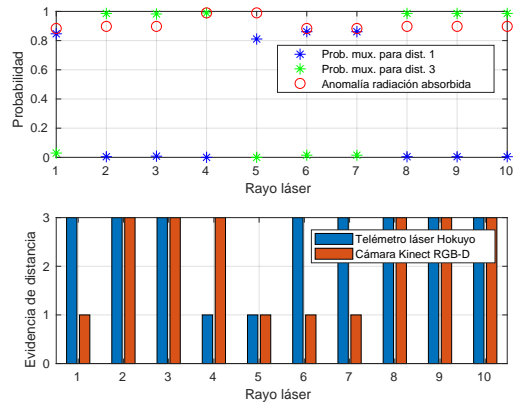
Figura 8: Resultados de inferencia para la prueba de anomalía de obstáculos negros. Se representan todos los rayos (horizontal) así como los datos de evidencia de los sensores reales (figura inferior) donde 1 corresponde a obstáculo no detectado y 2, 3... a obstáculos a distancias crecientes.
