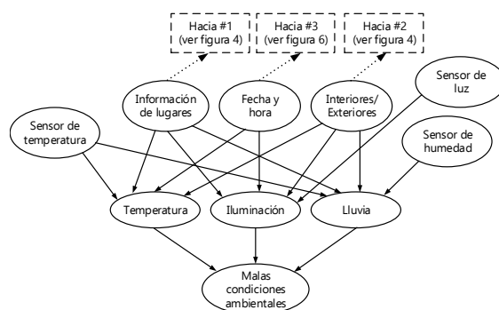
Figura 3: Detección de malas condiciones ambientales para la subred de anomalías.
