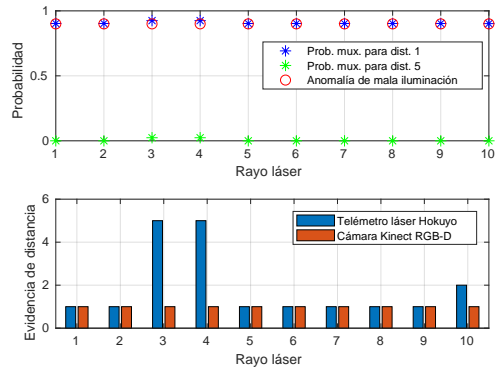
Figura 10: Resultados de inferencia para la prueba de anomalía por malas condiciones de iluminación. Se representan todos los rayos. Como recordatorio, la distancia 1 implica obstáculo no detectado, mientras que 5 corresponde a un rango discretizado de distancia de entre 3.3m a 4.4m.
