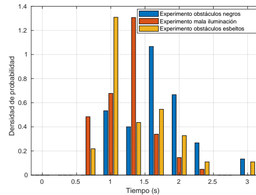
Figura 12: Distribuciones de probabilidad de los tiempos de ejecución para una iteración del bucle de control en todos los experimentos.
