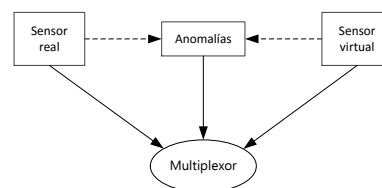
Figura 1: Sensor genérico basado en redes bayesianas. Se puede construir una arquitectura sensorial bayesiana completa interconectando elementos como éste a través de sus multiplexores.
