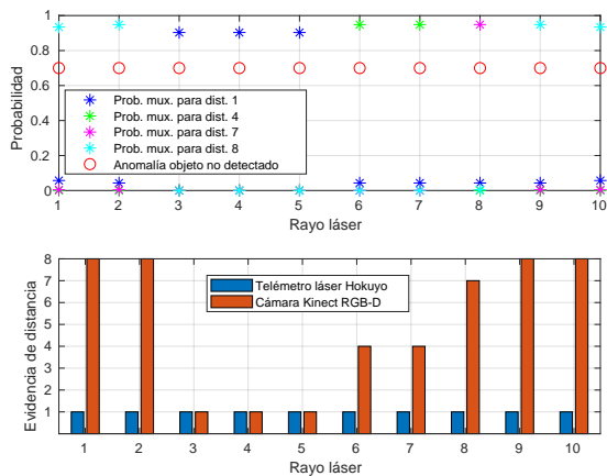
Figura 11: Resultados de inferencia para la prueba de anomalías por obstáculos esbeltos. El obstáculo se detecta mediante una distribución espacial más fina de los rayos láser. De nuevo, la distancia 1 significa que no se ha detectado obstáculo.
