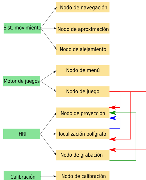
Figura 2: Diagrama de bloques del sistema propuesto. Los cuatro bloques principales (verde) están compuestos por uno o varios nodos ROS (naranja) que se comunican entre sí para permitir al robot jugar con el usuario.
