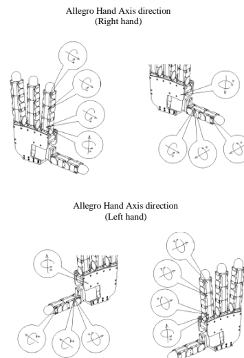
Figura 2: Rotación de las articulaciones de la mano Allegro
