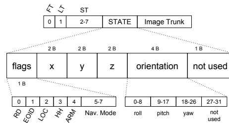
Figura 7: Mensaje que transmite el ROV
