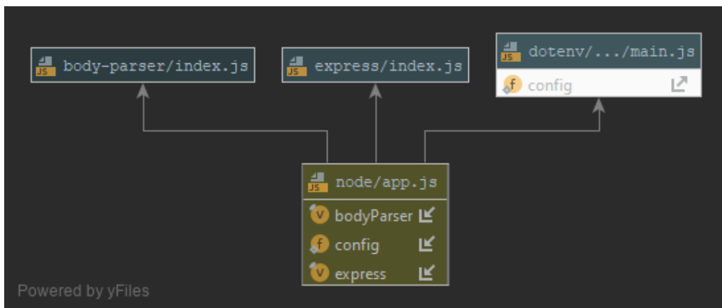
Ilustración 28 – Diagrama UML del módulo de red (JavaScript)
