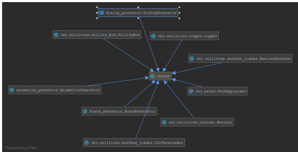
Ilustración 32 - Diagrama UML del módulo de utilidades
