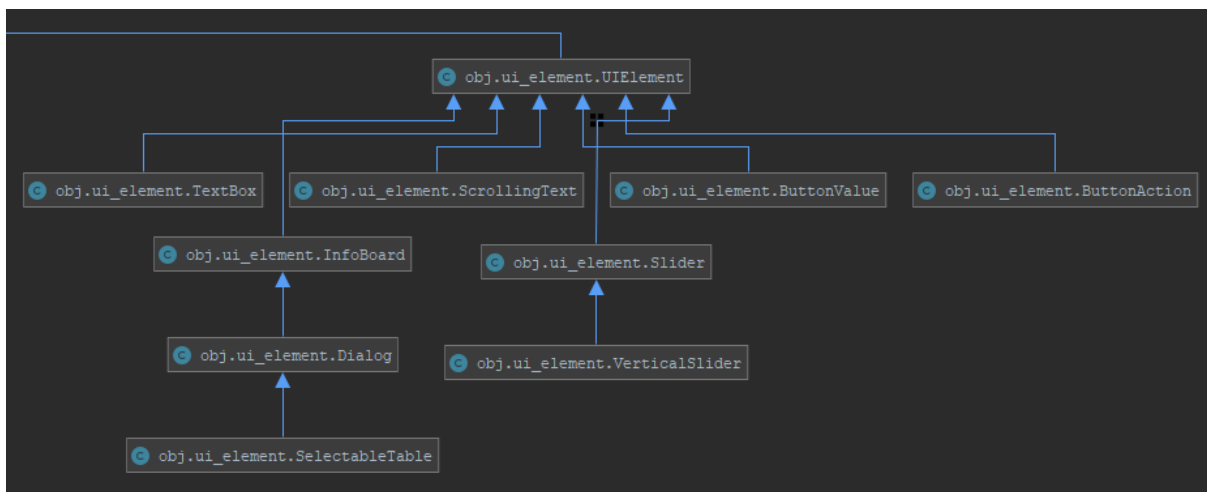
Ilustración 26 - Diagrama UML del módulo gráfico (Solo UIElement)
