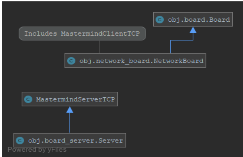
Ilustración 27 – Diagrama UML del módulo de red (Python)
