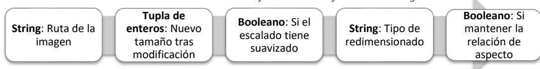
Ilustración 35 - Atributos de un objeto ResizedSurface de una imagen
