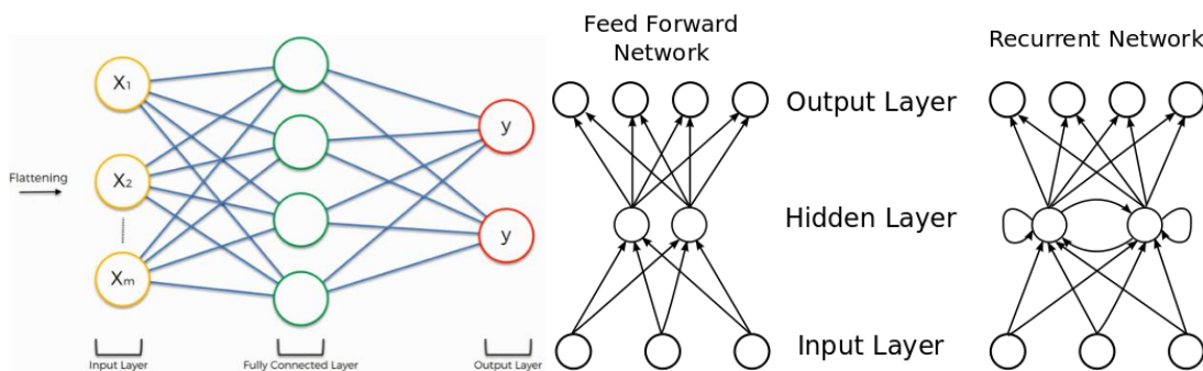
Ilustración 7 y 8 – Izquierda: RN Convolutiva, Centro: RN Prealimentada, Derecha: RN recurrente
