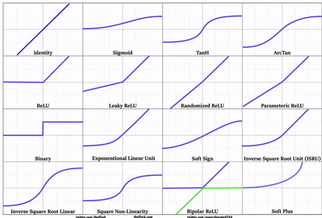
Ilustración 9 – Representación gráfica de funciones de activación (Animado en Link fuente).
