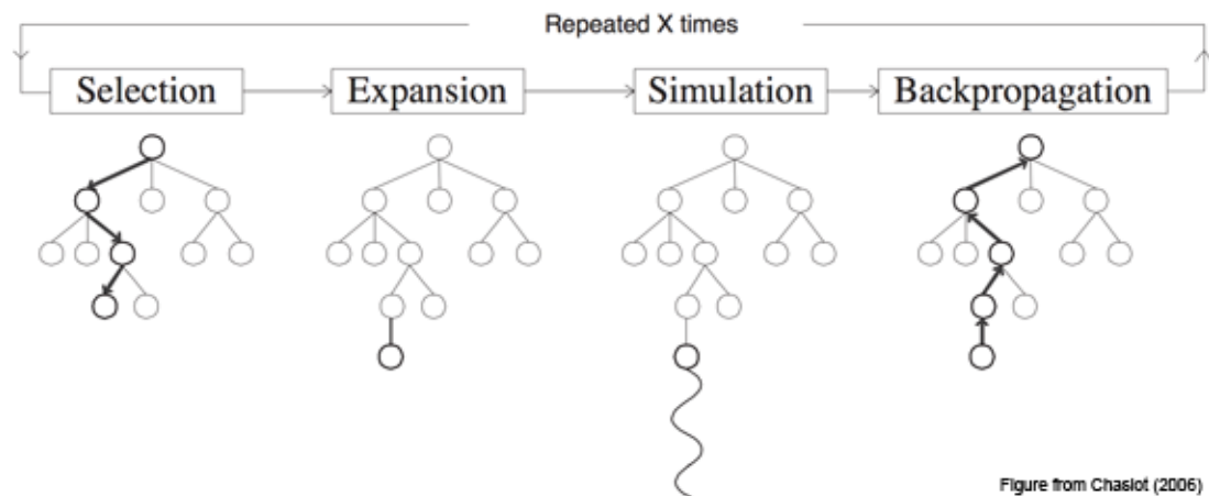
Ilustración 45 – Representación gráfica proceso del MCTS
