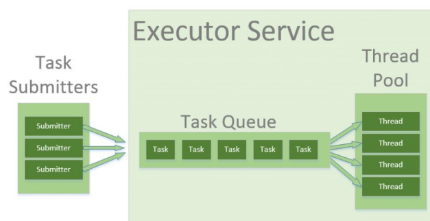
Ilustración 37 – Representación gráfica del proceso (Agrupamiento de hilos)
