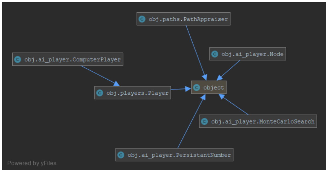
Ilustración 29 - Diagrama UML del módulo de IA
