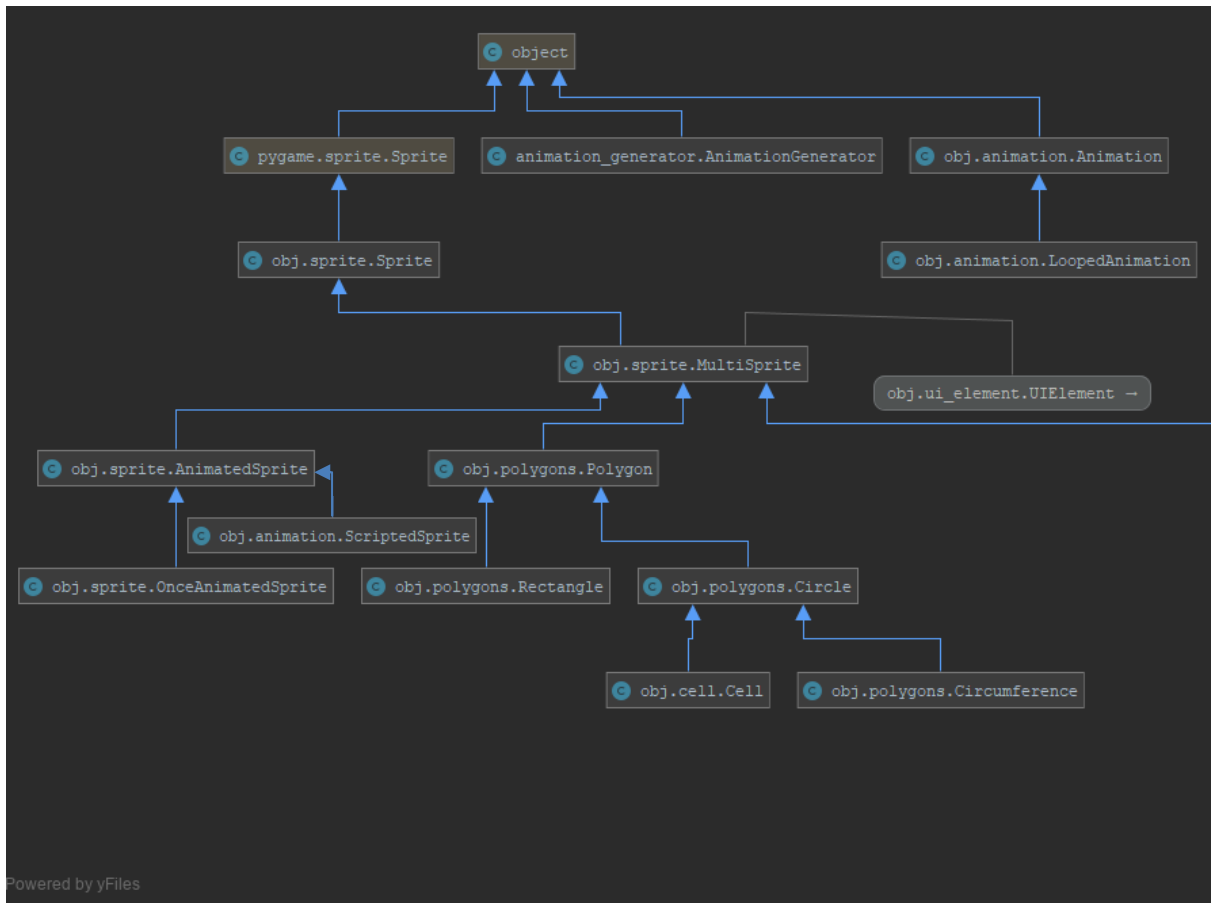
Ilustración 25 – Diagrama UML del módulo gráfico (Excepto UIElement)
