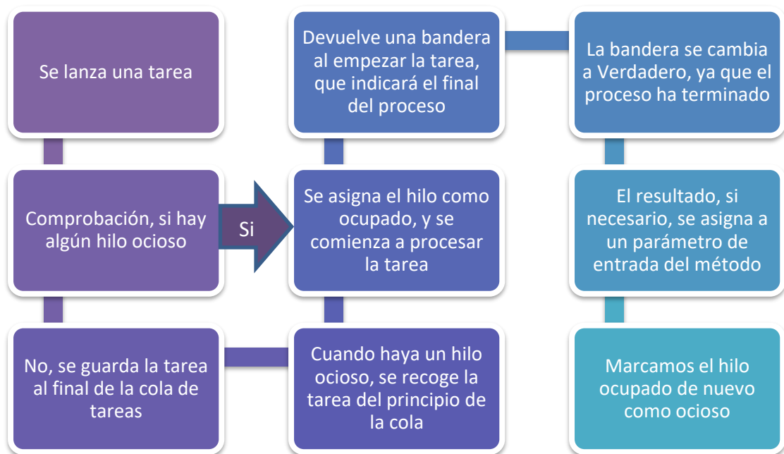
Ilustración 36 - Flujo de paso de las tareas mediante Thread Pooling
