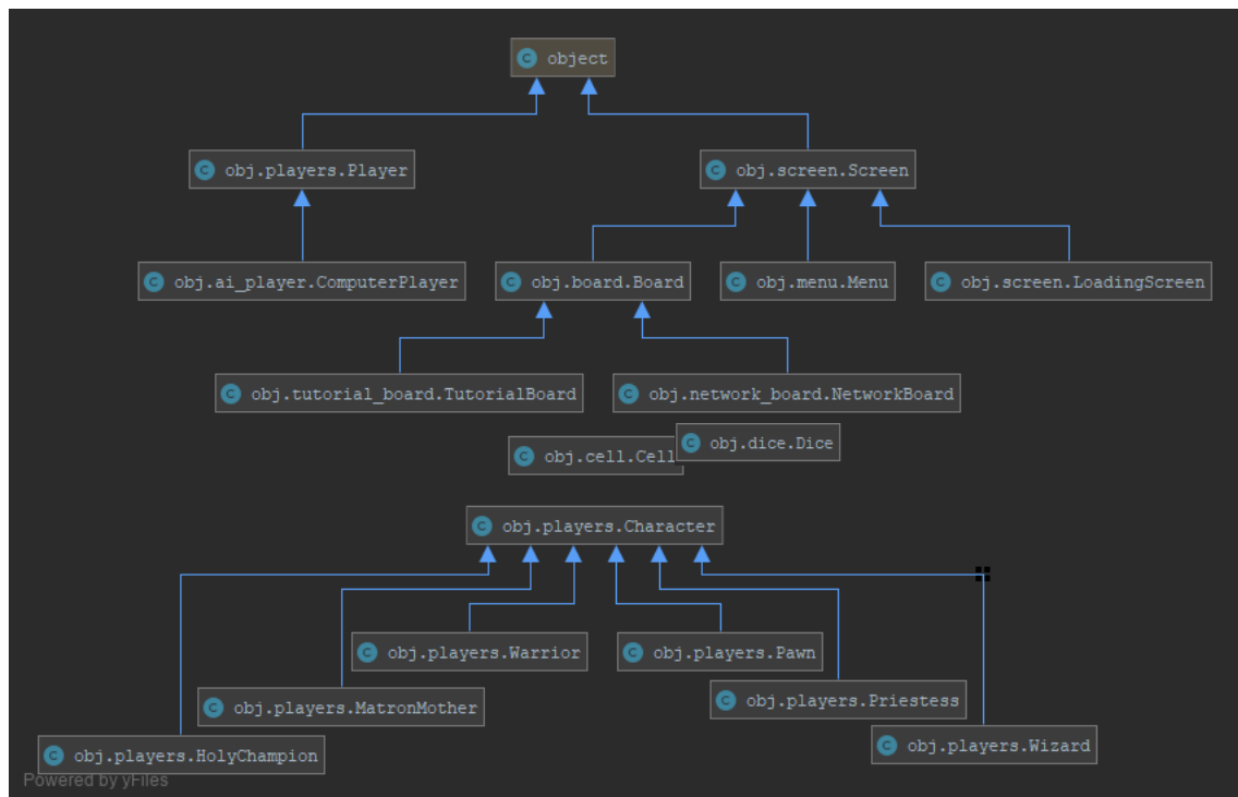
Ilustración 30 - Diagrama UML del módulo de interacción
