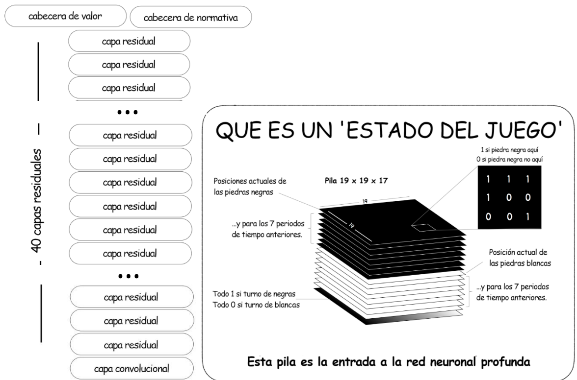
Ilustración 17 – Estado del juego, AlphaGo
