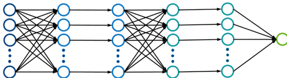
Ilustración 6 – Red neuronal con dos capas totalmente conectadas (1ª y 3ª)
