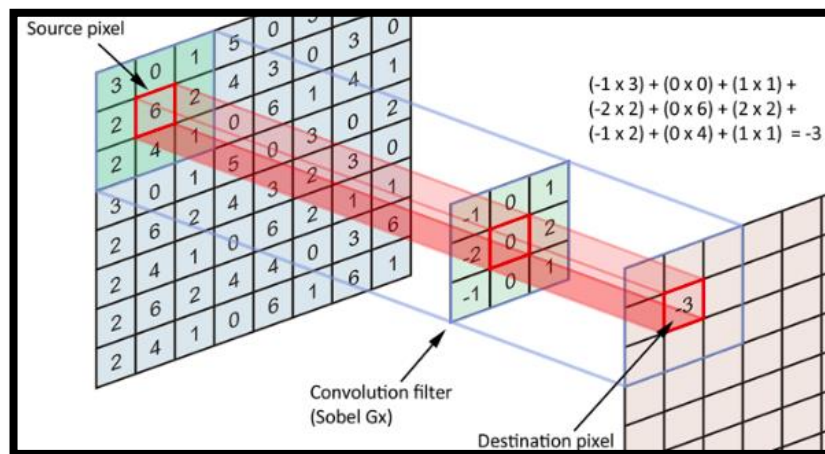
Ilustración 5 – Diagrama de una convolución
