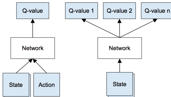
Ilustración 11 – Izquierda: Esquema básico de una Red profunda-Q, Derecha: Arquitectura más optimizada
