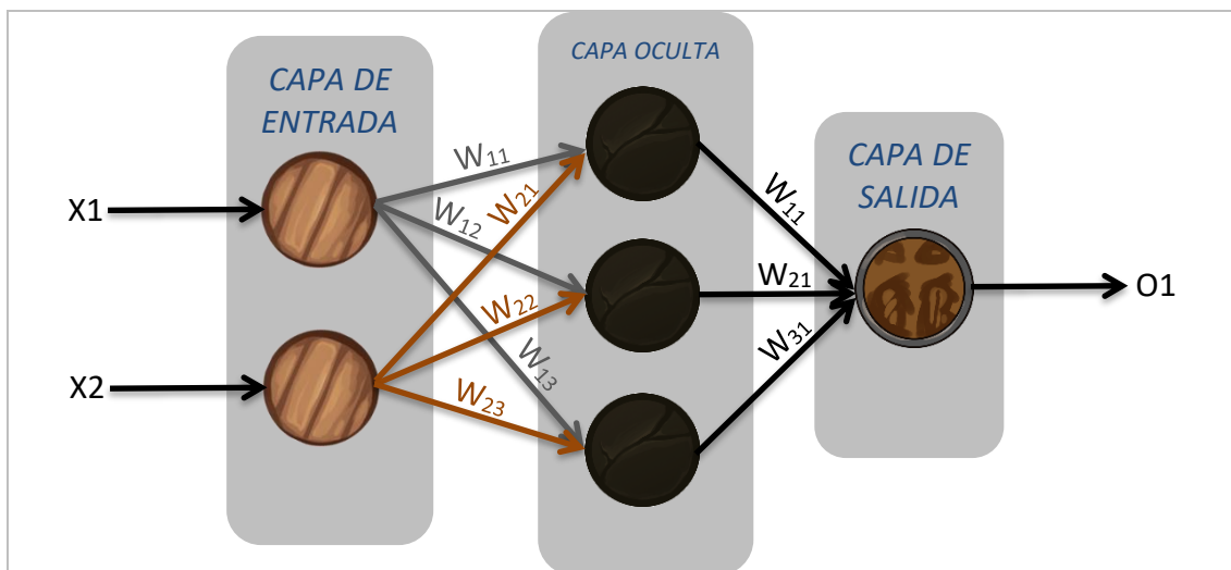
Ilustración 2 – Perceptron Multicapa
