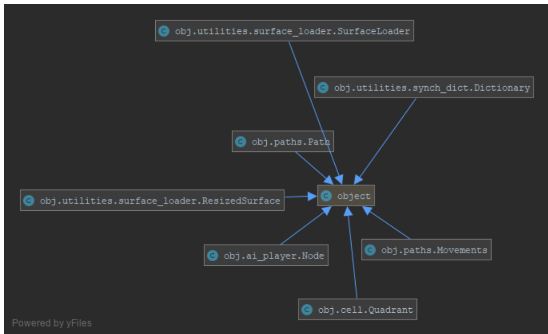
Ilustración 31 - Diagrama UML del módulo de estructuras
