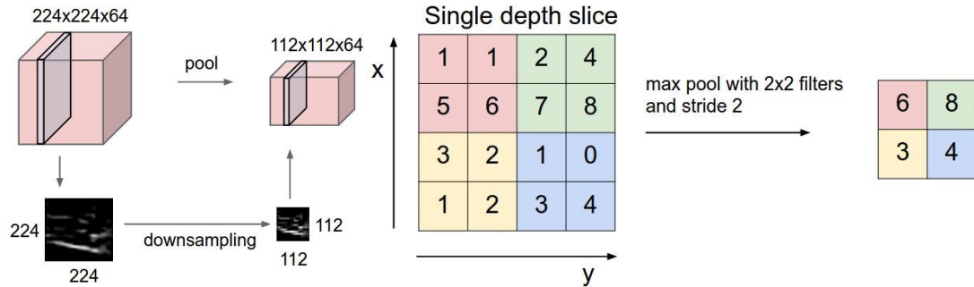
Ilustración 4 – Salida de una capa de agrupación
