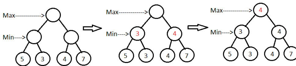
Ilustración 43 – Ejemplo de ejecución MiniMax
