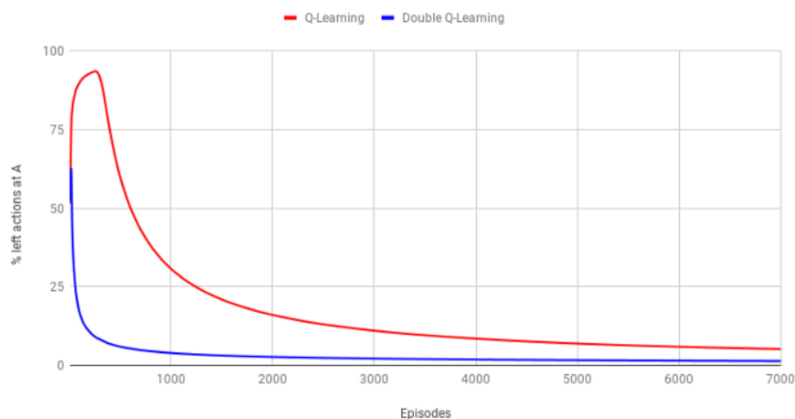
Ilustración 12 – Comparación de rendimiento en un entorno con 100 acciones posibles.
