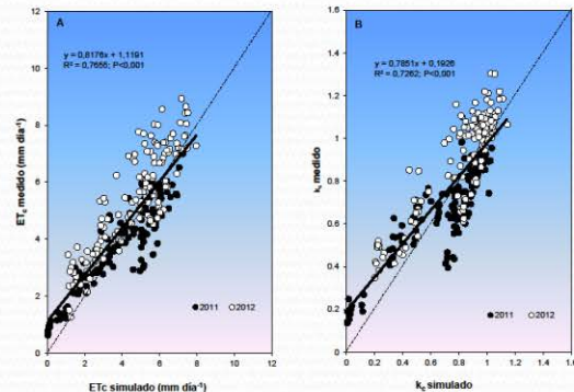
Figura 2. Relación lineal entre los valores de ET_c (A) y k_c (B) simulados mediante CS y medidos en campo durante los años 2011 y 2012.
