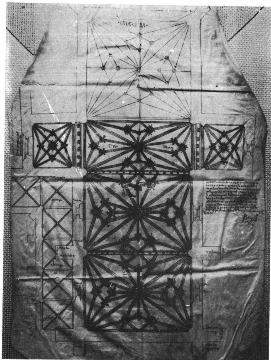
Lám. 1. CATEDRAL DE CORIA: Traza de Bartolomé de Pelayos
