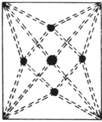
Fig. 10. Catedral de Coria, Bóveda de brazo del crucero (Proyecto de B. de Pelayos)
