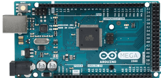
Fig. 5.1: Arduino Mega
