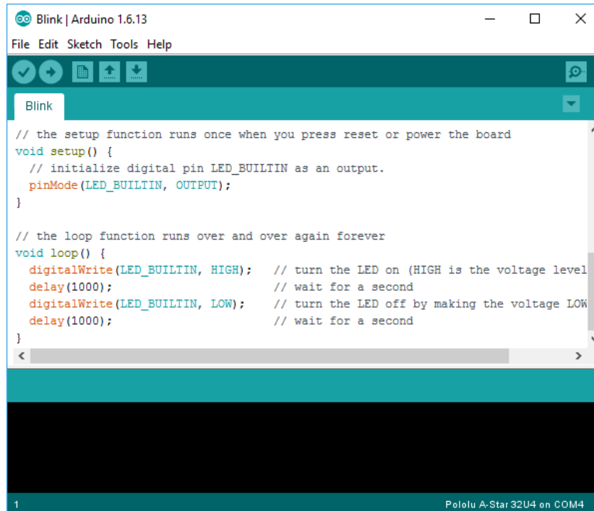
Fig. 5.7: Arduino IDE
