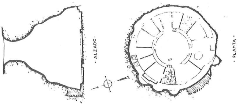
Granada — Alhambra. Planta y sección de la mazmorra de la Alcazaba
