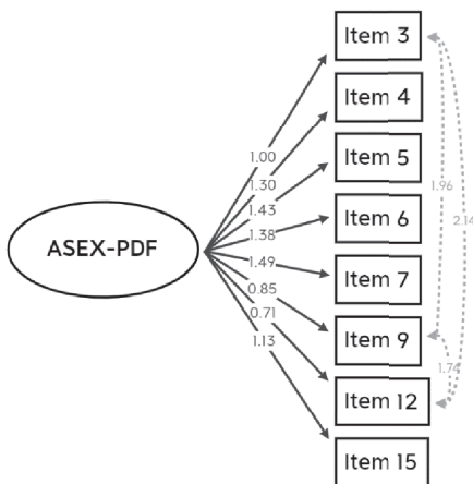
Fig. 1 Diagrama de ruta del modelo unifactorial
