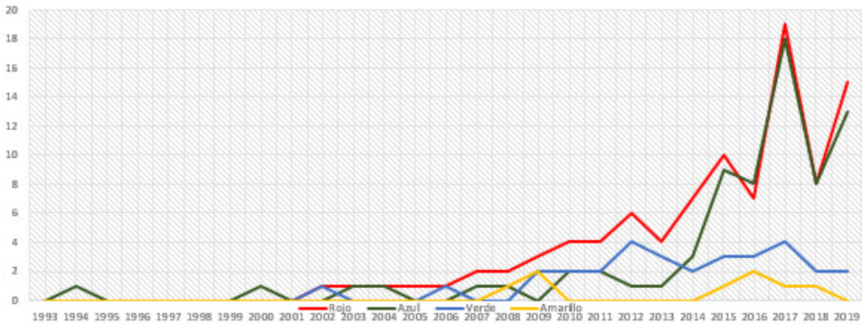
Figura 4. Tendencia por clúster en el desarrollo de las investigaciones en “DI” e “ICT”.
