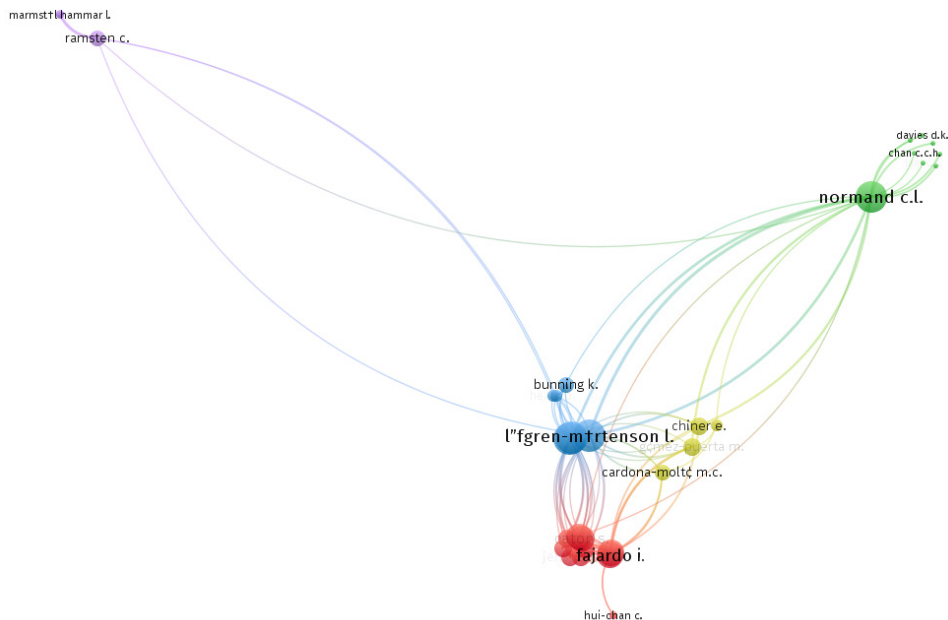
Figura 6. Autores que son mayormente citados en temas de "DI" e "ICT".
